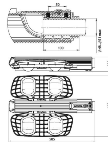
Рисунок 3. Габаритный чертеж
